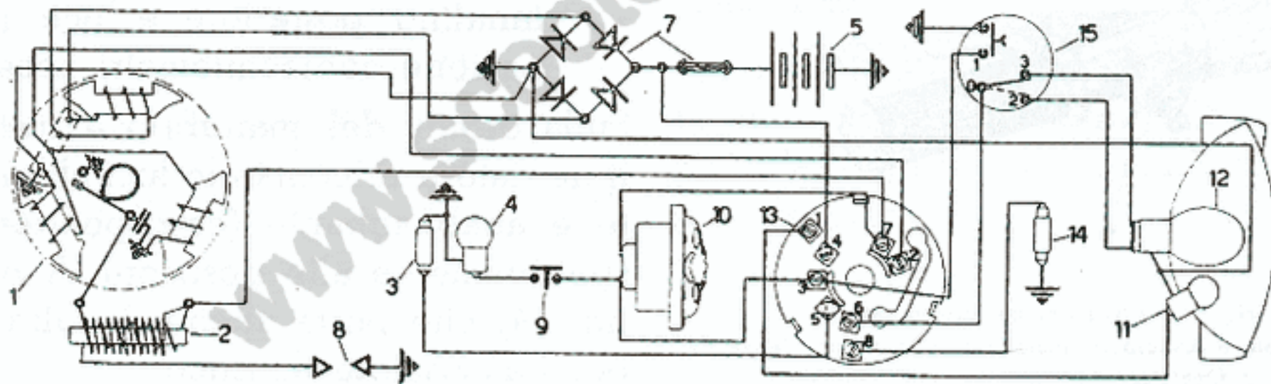
Fig. 13 - Collegamenti e schema elettrici
