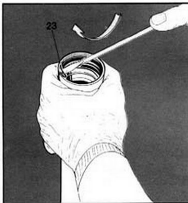
FIG. 8 Per togliere l'anello di tenuta (22) dal portaruota occorre togliere l'anello di fermo (23) con un cacciavite (rif.5) col quale si eserciterà una pressione sotto di esso.
