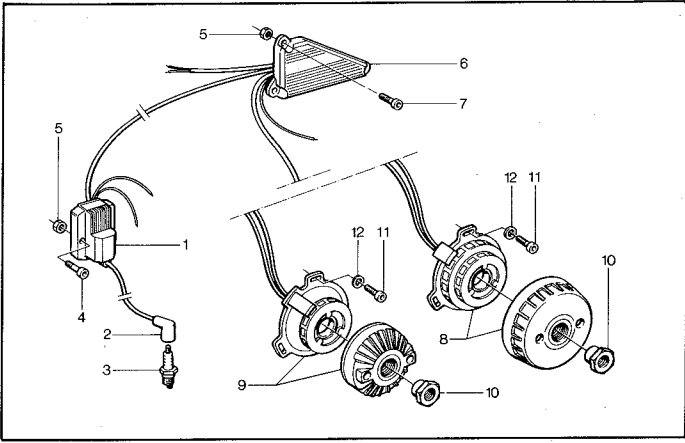
Tändsystem. Ignition.
