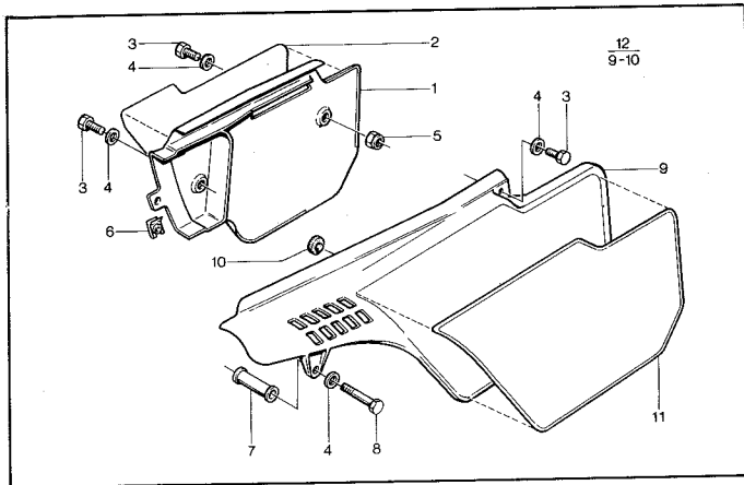
Sidopaneler. Sidecovers.
