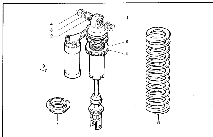
Stötdämpare. Shockabsorber.
