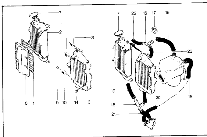
Kylare. Radiators.
