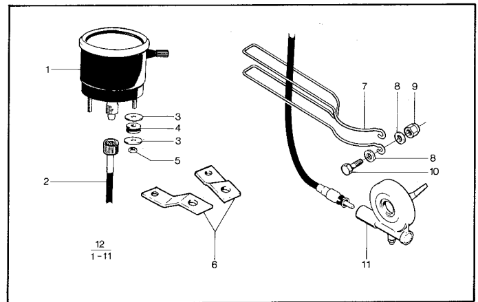
Hastighetsmätare. Speedometer.
