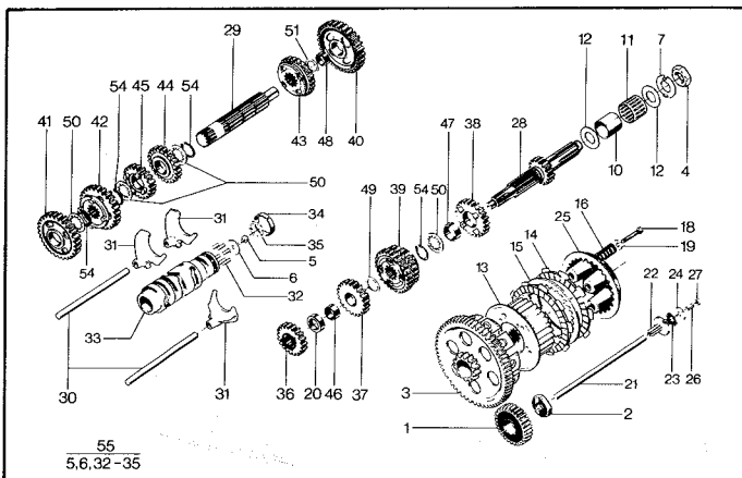
Växellåda. Gearbox.
