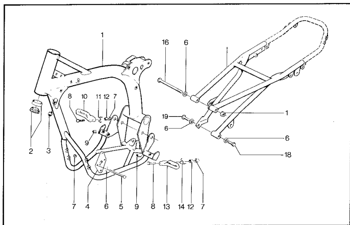
Ram. Frame.
