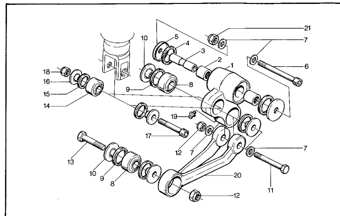
Stötdämparlänkage. Shocklinkage.
