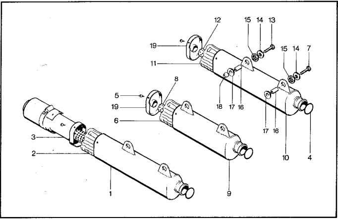
Ljuddämpare. Silencer.
