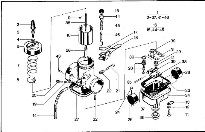
Förgasare. Carburettor.
