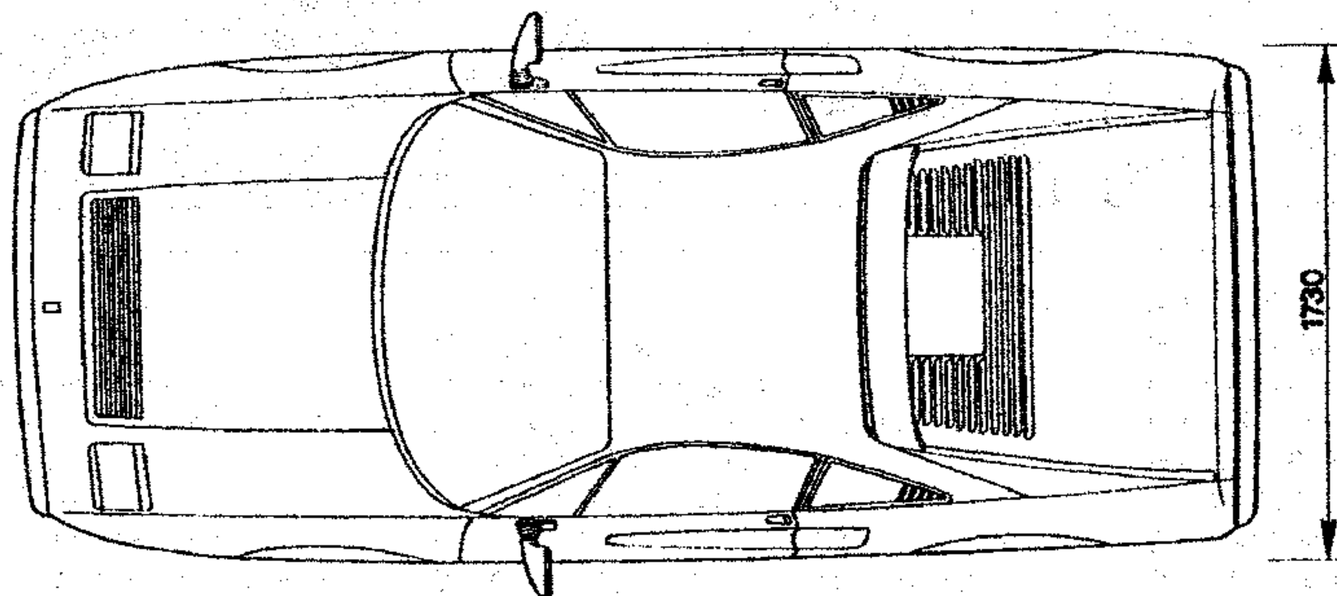
Fig. 2 = Ingombro vettura 328
