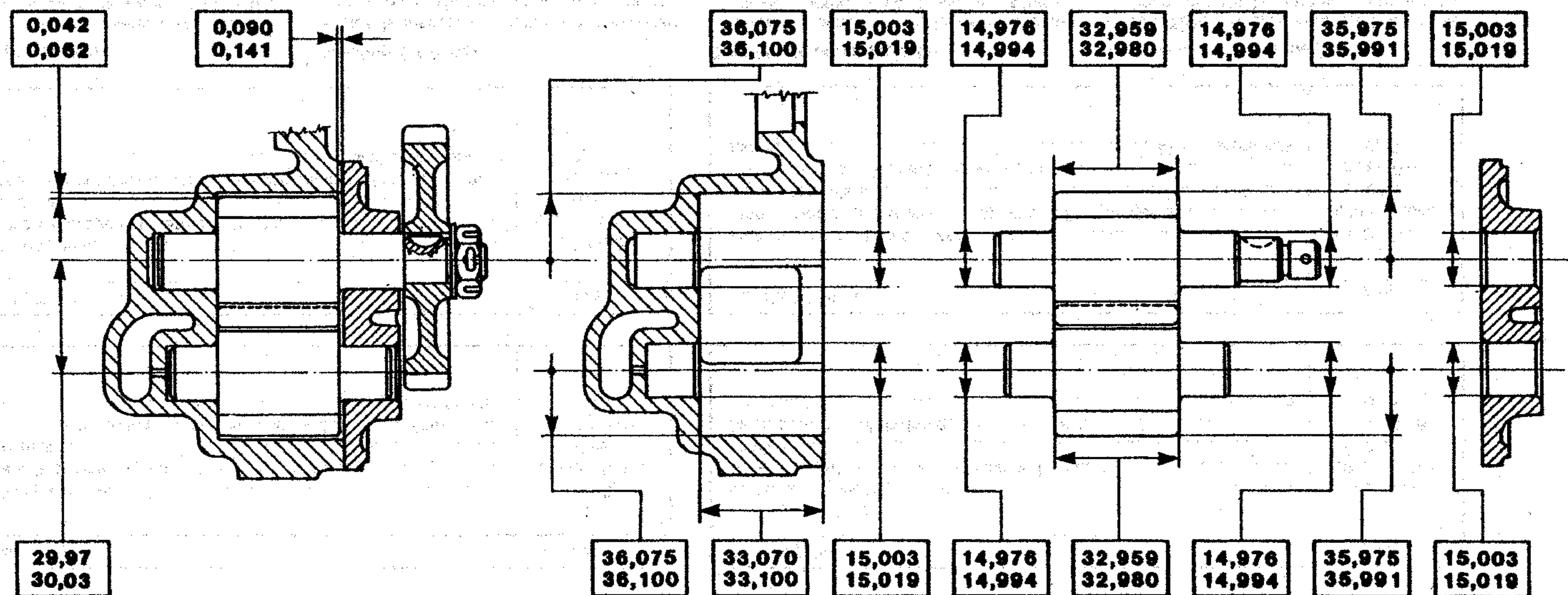
Fig. 2 = Pompa olio
