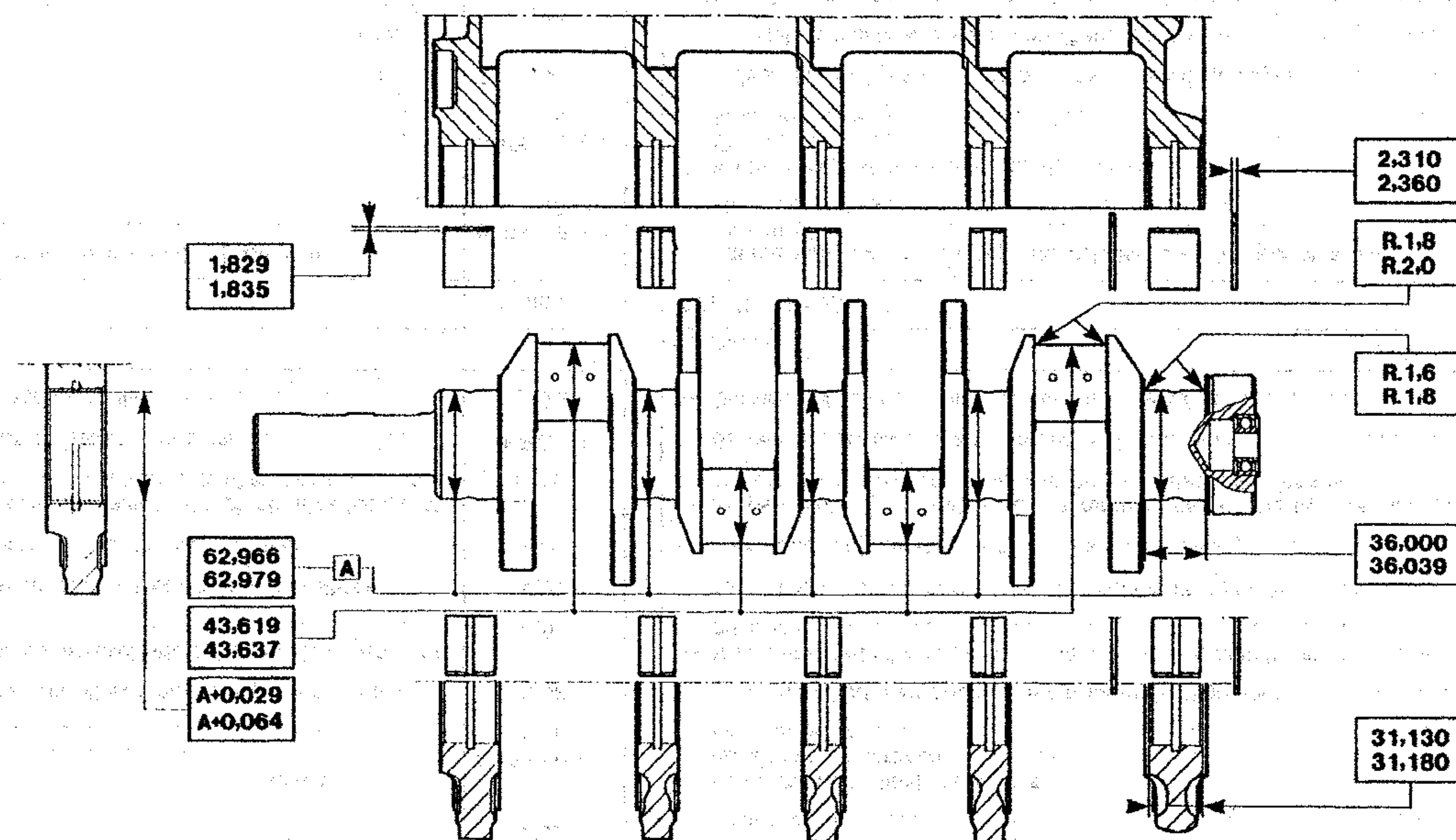
Fig. 9 = Albero motore
