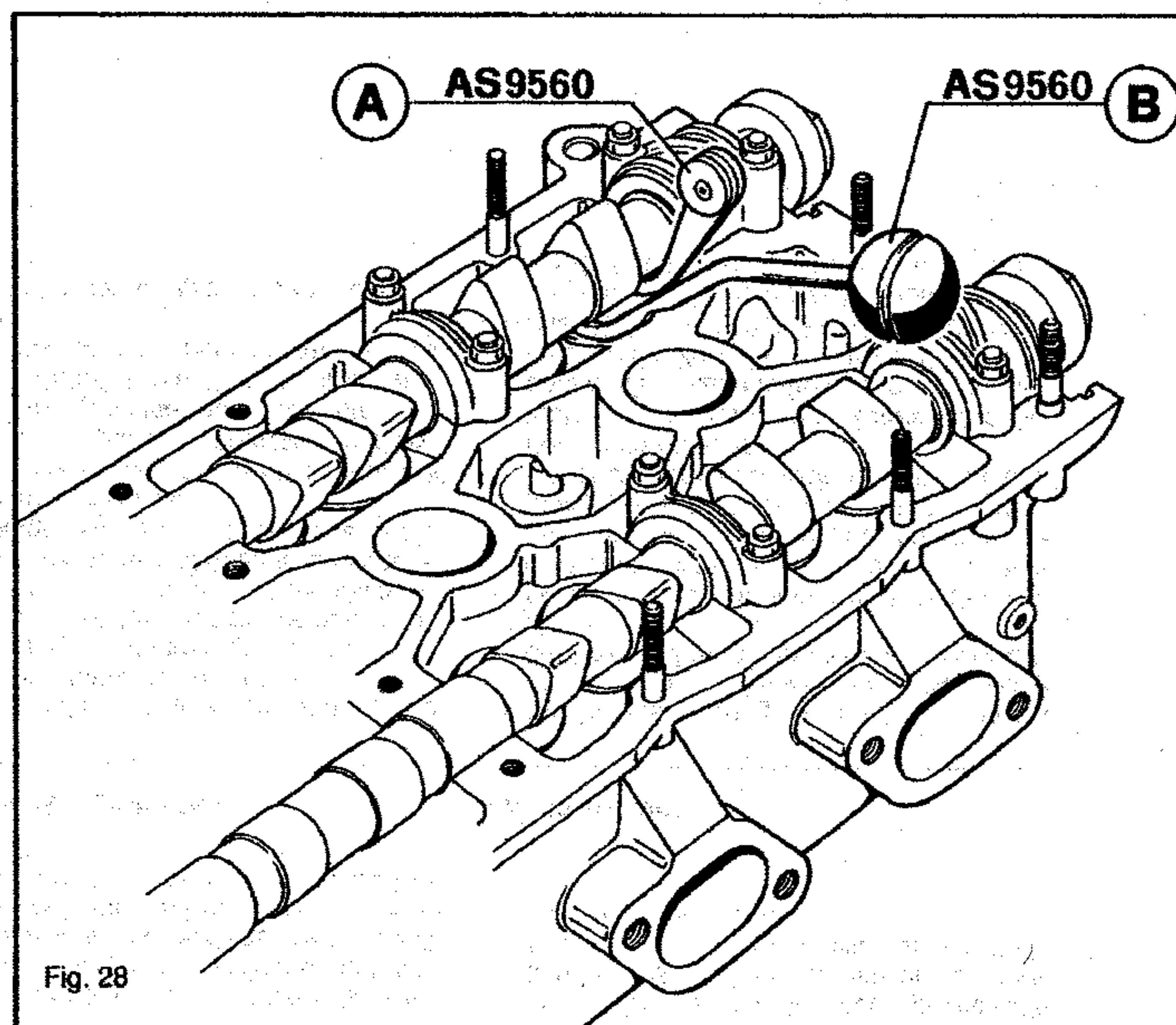
Fig. 27 = Contrôle du jeu Fig. 28 = Démontage des pastilles
