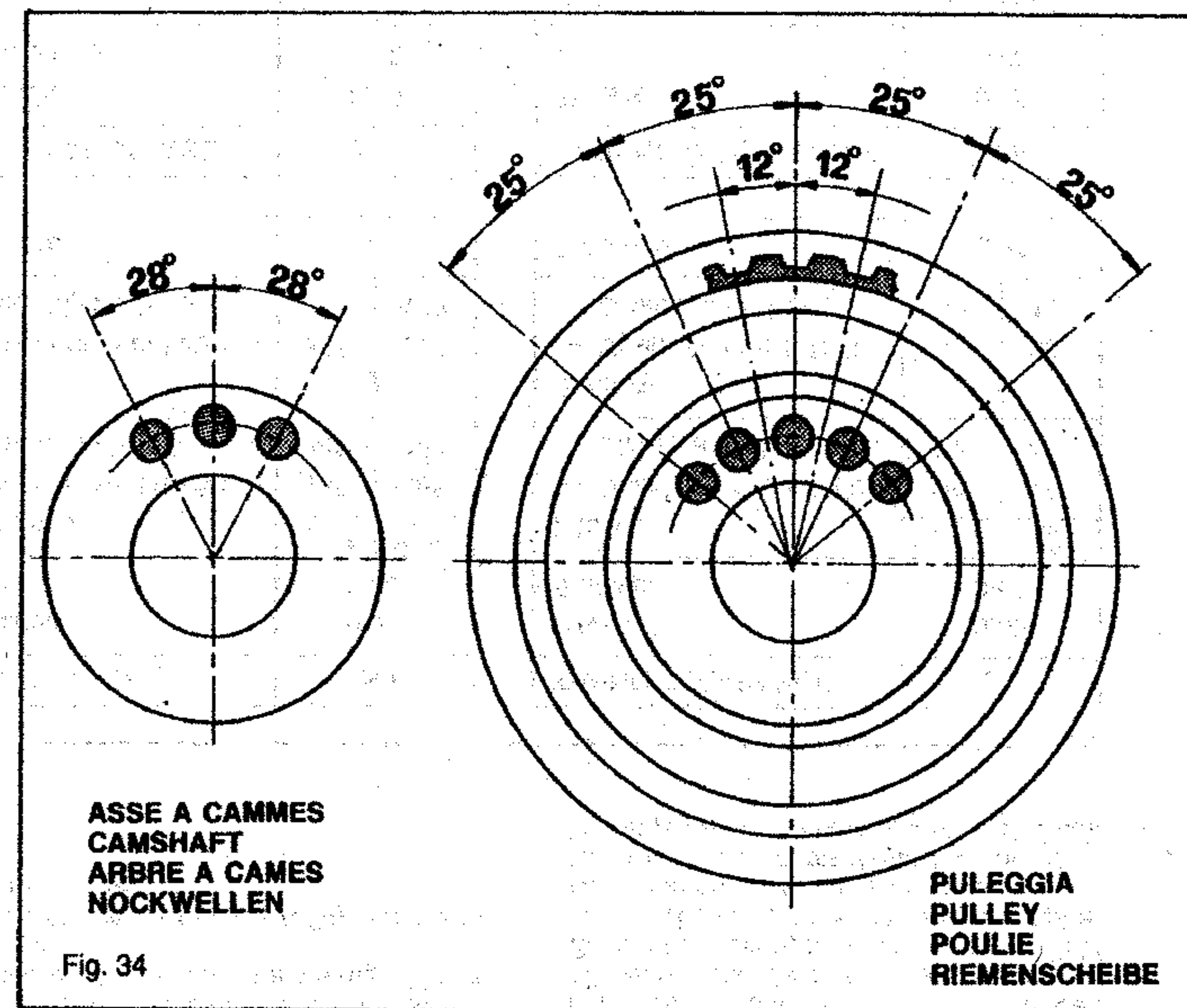
Fig. 33 = Tendeur de courroie A = Ecrout de réglage Fig. 34 = Trous de poulies et des arbres à cammes
