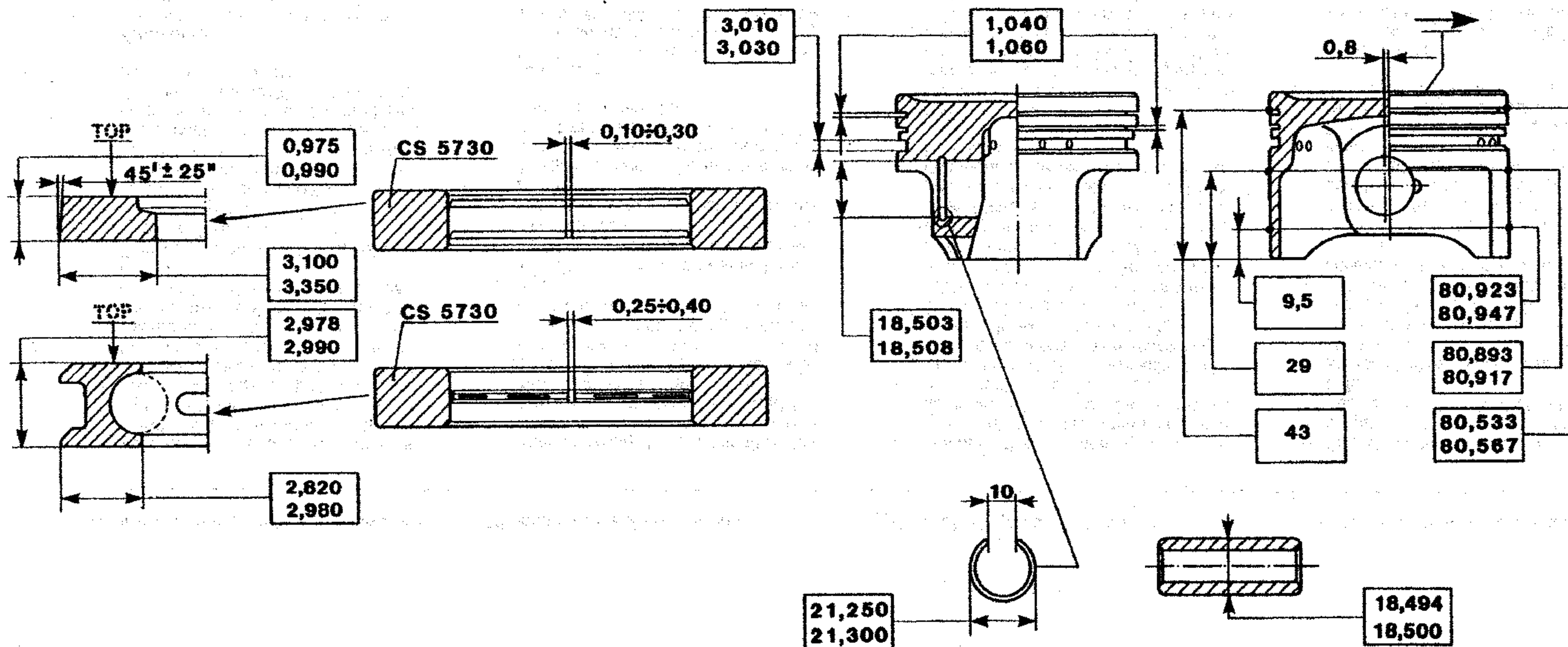
Bild 11 = Kolben und Kolbenringe Hauptdaten
