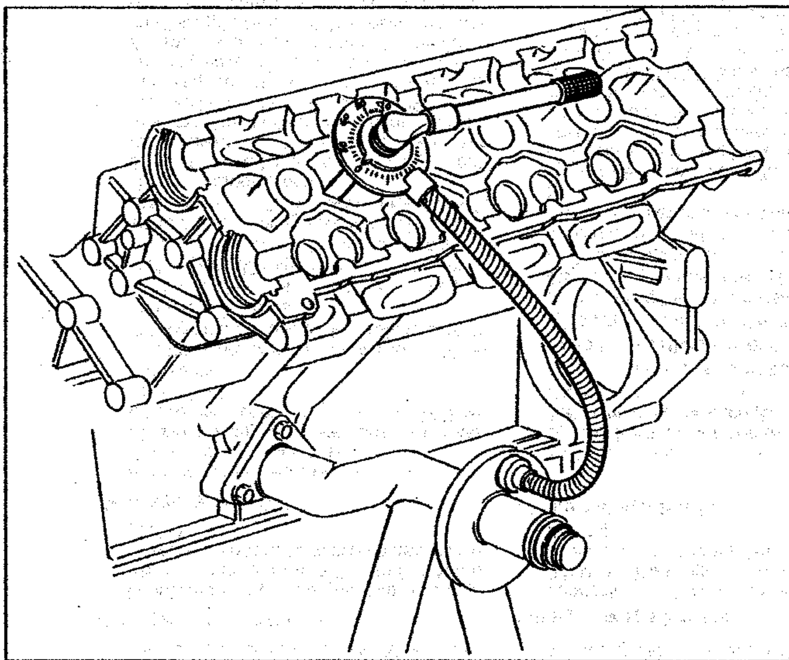
Fig. 40 = Serraggio teste con atrezzo USAG 830
