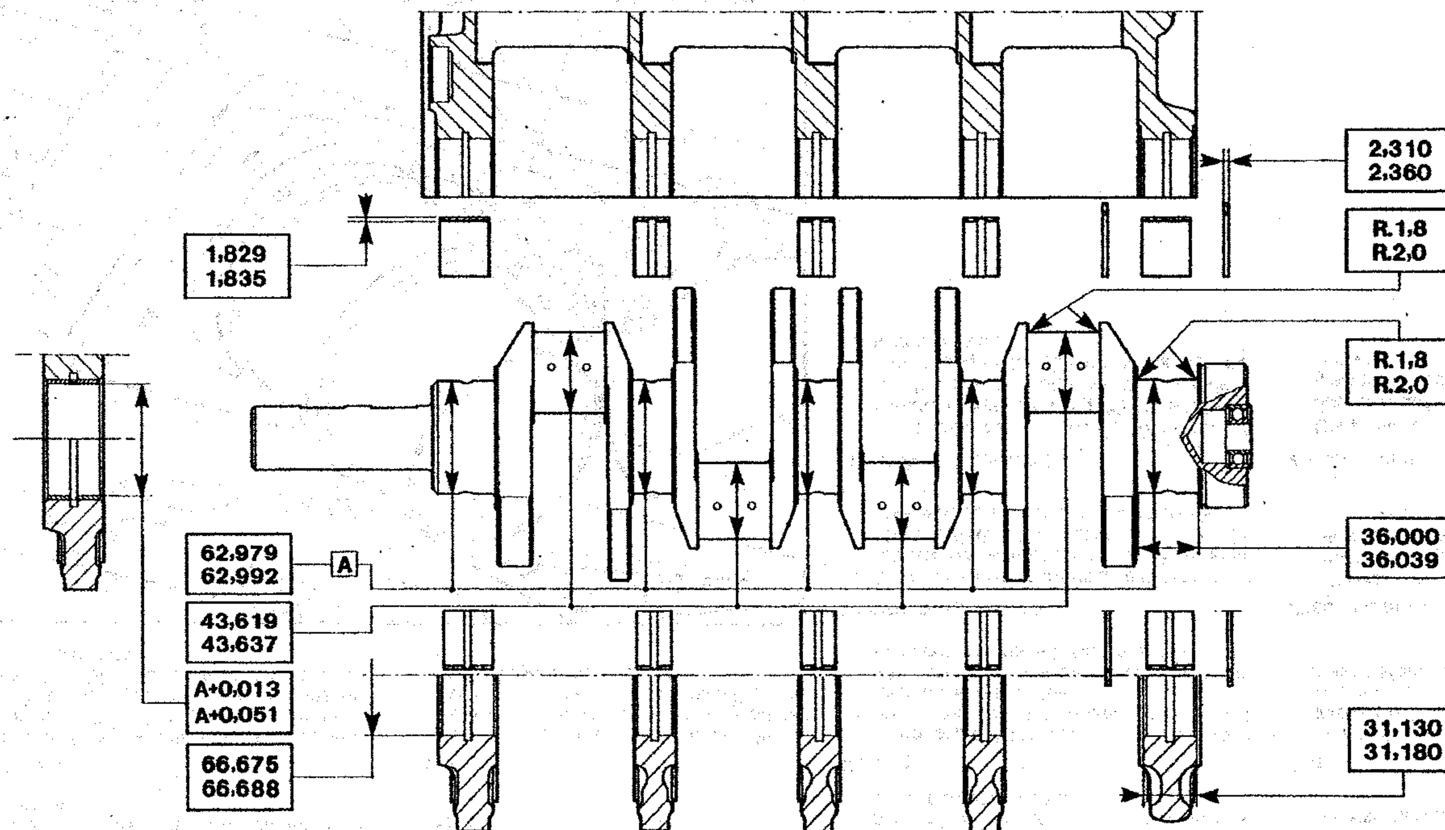
Fig. 39 = Albero motore
