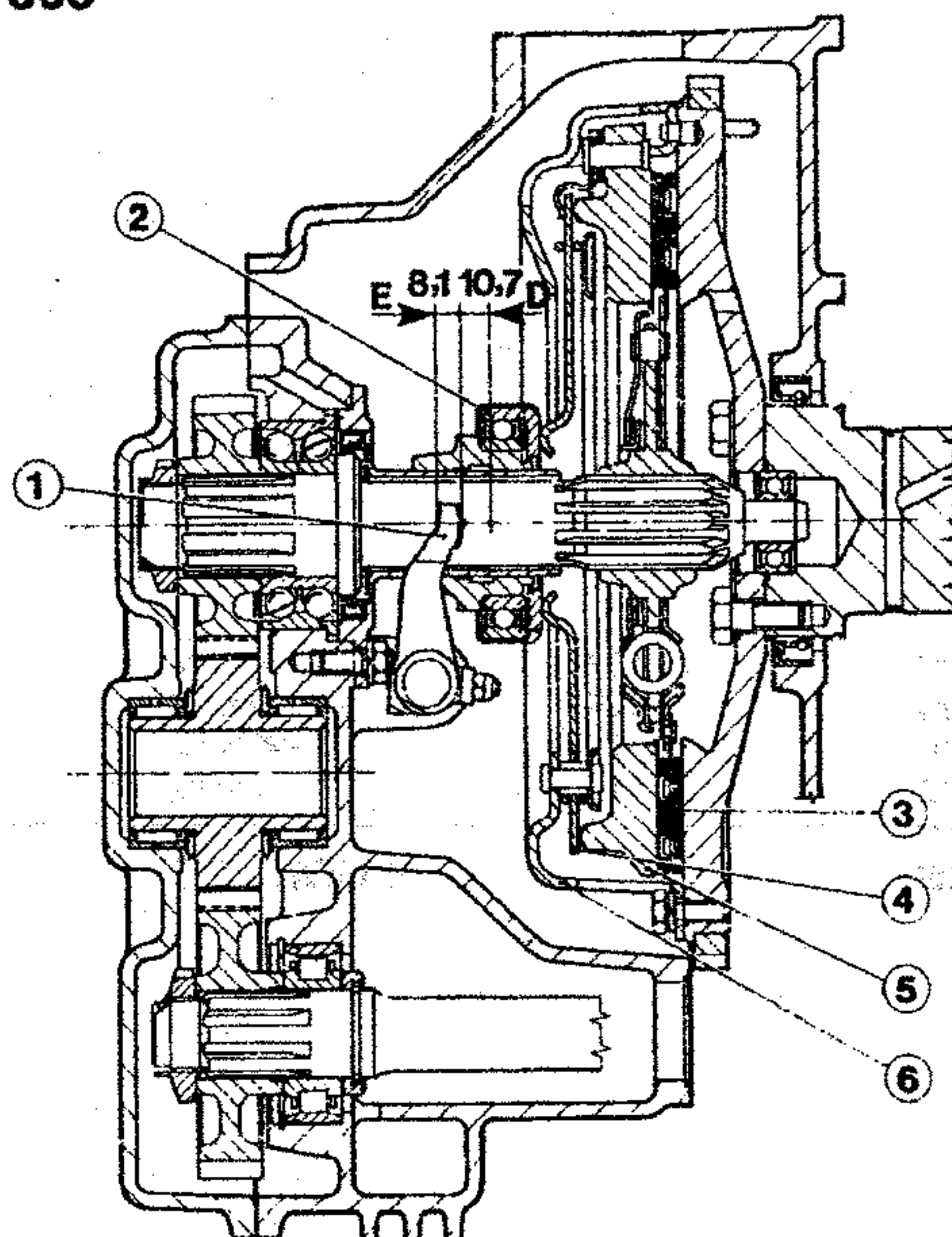
Bild 1 = Kupplung und Kupplungs-Nehmerzylinder
