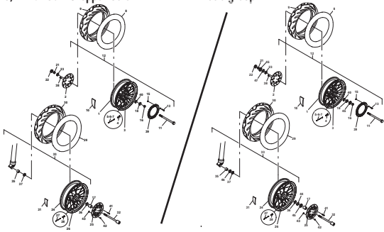
TAV.15/ TAV. 15a- Gruppo ruote - Wheels group M4
