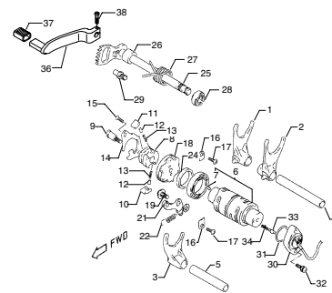
TAV.8 - Cambio velocità - Gear box
